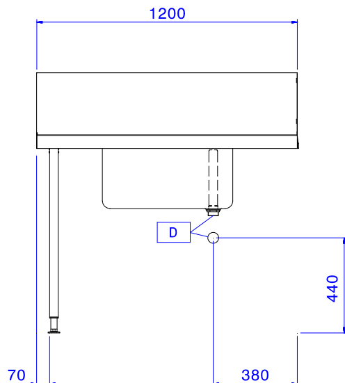
Front aanzicht
